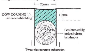
Figuur 2: Ondiepe voeg.
